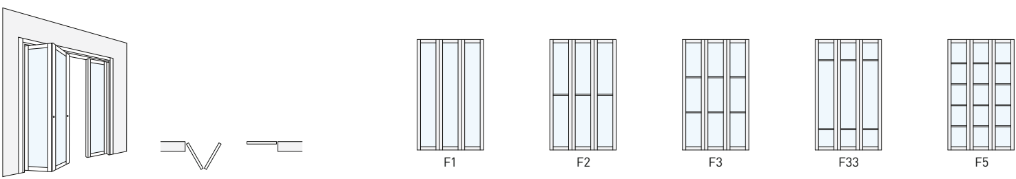
Porta a libro a tre ante (di cui una semi-fissa) / three-wing centre split folding doors (one semi-fixed wing)
