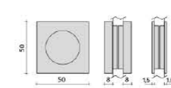
Maniglia quadrata ad incasso Escluso Synthesy Stylo e Quadra Recessed square handle Not available on Synthesy Stylo e Quadra
