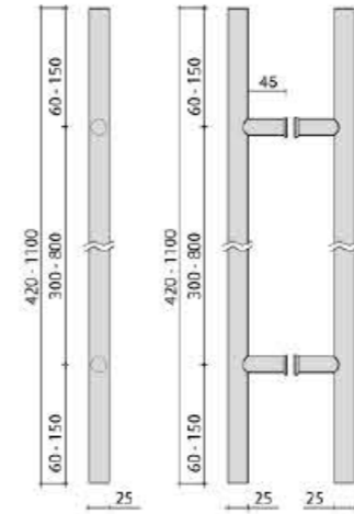
MD/420 - MD/1100 Maniglione doppio altezza mm 420/1100 Double pullhandle height 420/1100 mm
